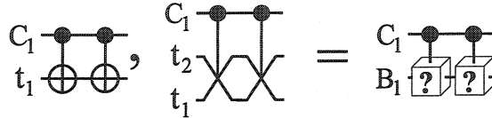
Figure 5.4: Class AA.
