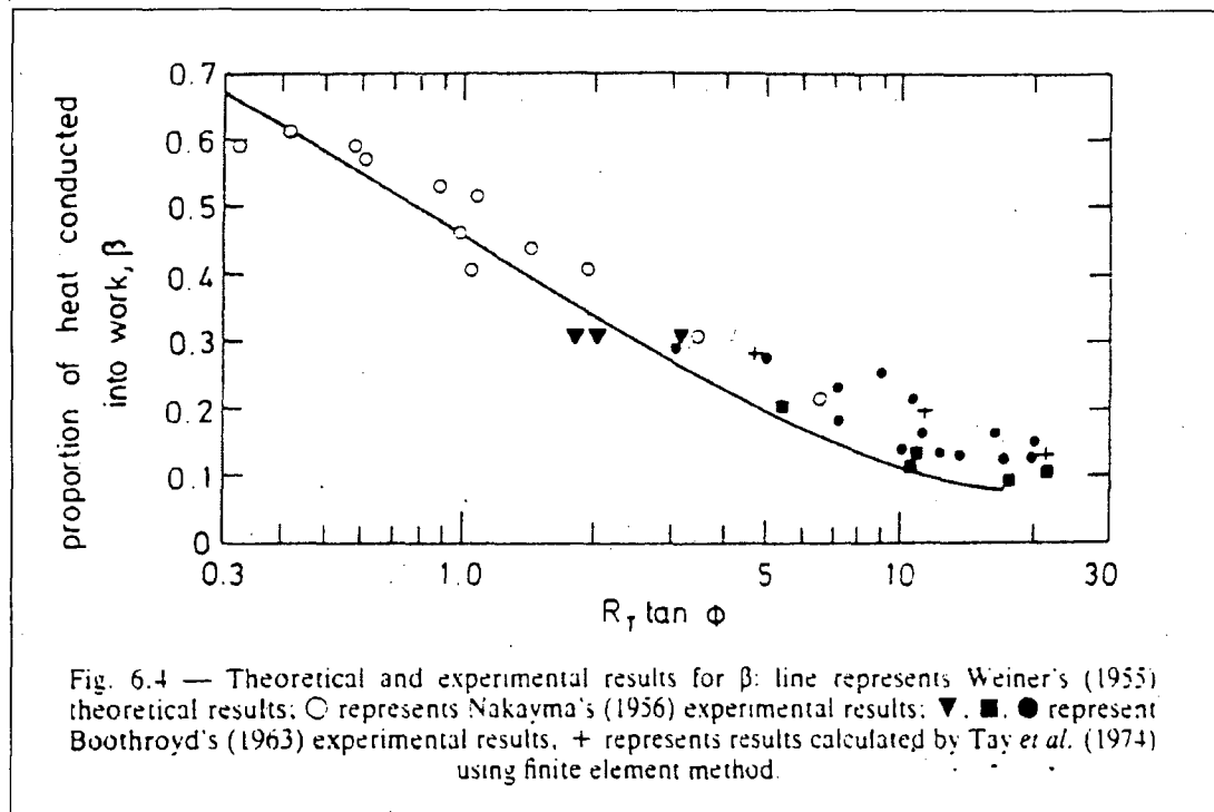
Figure 1.17 Estimation du coefficient \xi^7 [9].
