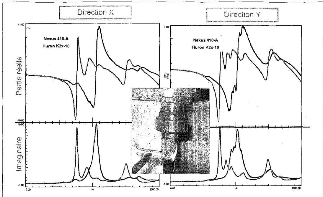
Figure 3.5 Fonctions de transfert (FRF) de deux machines-outils.
