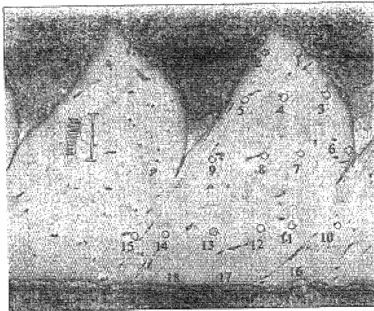
Figure 2-26 : Valeurs de dureté relevées sur un copeau d'acier austénitique nuance U ( V_c=150 m/min, a=0,3 mm/tr, outil carbure, angle de coupe 5^\circ ). Le point 6, trop au bord, n'est pas retenu.
