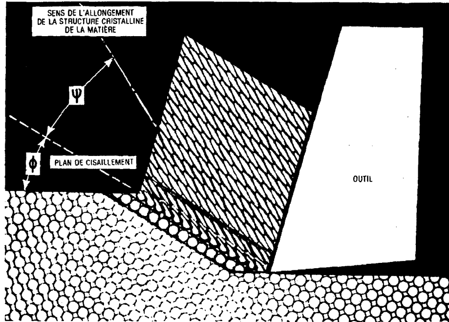
Figure 1.12 Détermination de l'angle \psi à partir de la déformation de la structure cristalline de la matière sur une micrographie [7].
