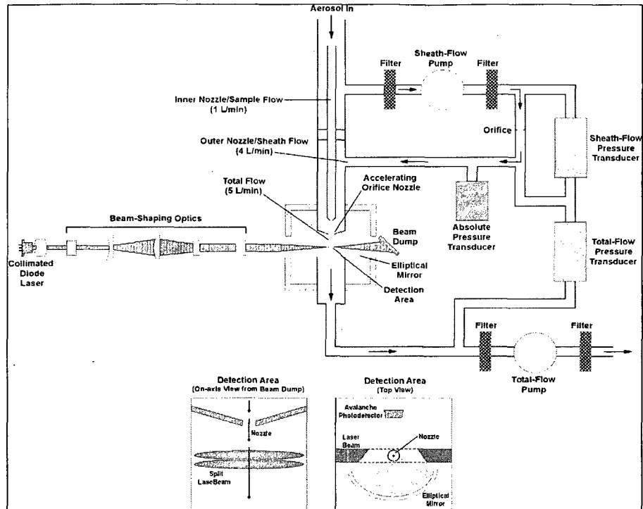
Figure 3.1 Schéma descriptif de l'APS ( http://www.tsi.com ).
