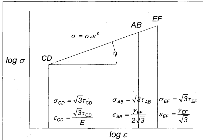
Figure 2.5 Graphique pour obtenir le coefficient d'érouissage \eta définie par l'équation 2.9.
