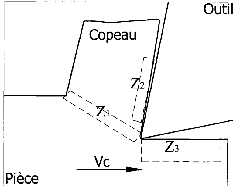
Figure 2.4 Les trois zones de cisaillement.
