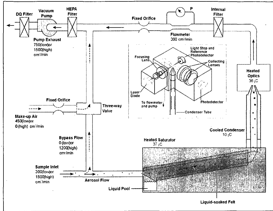
Figure 3.2 Schéma descriptif de CPC ( http://www.tsi.com ).
