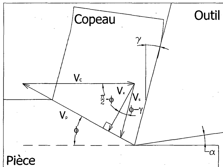
Figure 1.10 Diagramme des vitesses.
