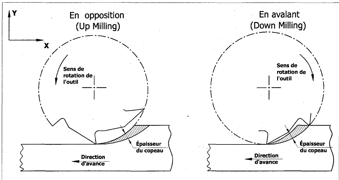
Figure 1.2 Fraisage en avalant et en opposition.
