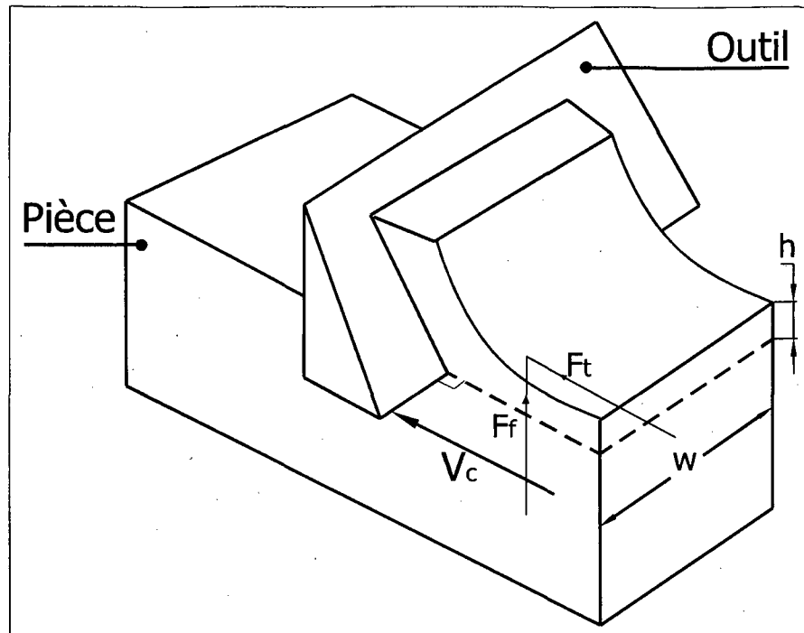
Figure 1.4 Géométrie de la coupe orthogonale.
