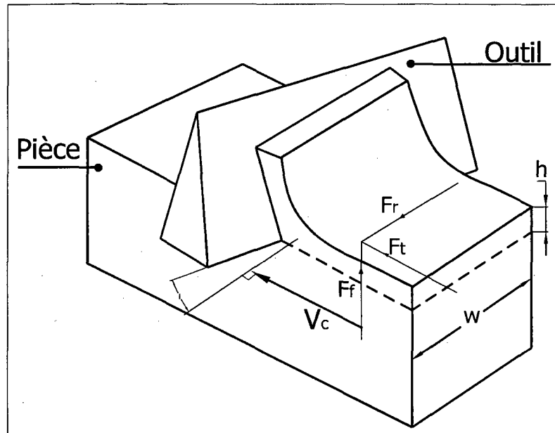
Figure 1.5 Géométrie de la coupe oblique.
