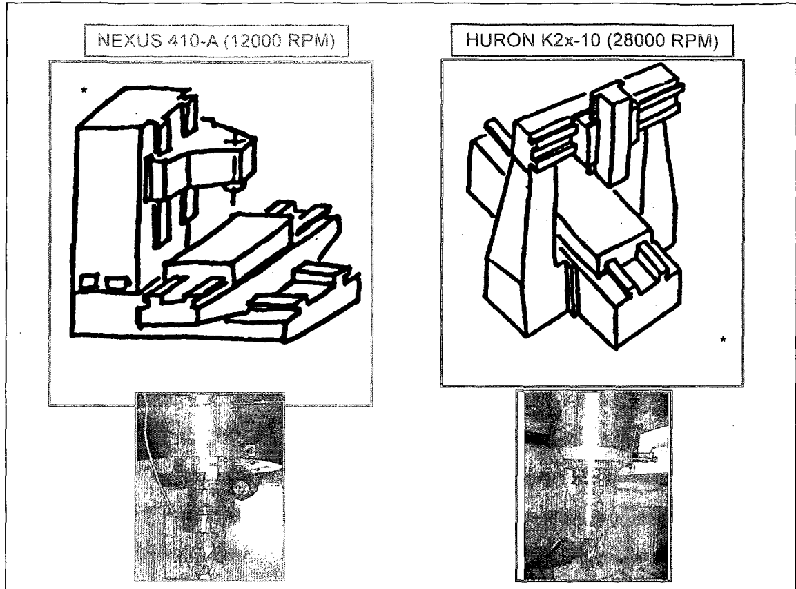
Figure 3.4 Structure générale de deux machines-outils (* Source [13]).
