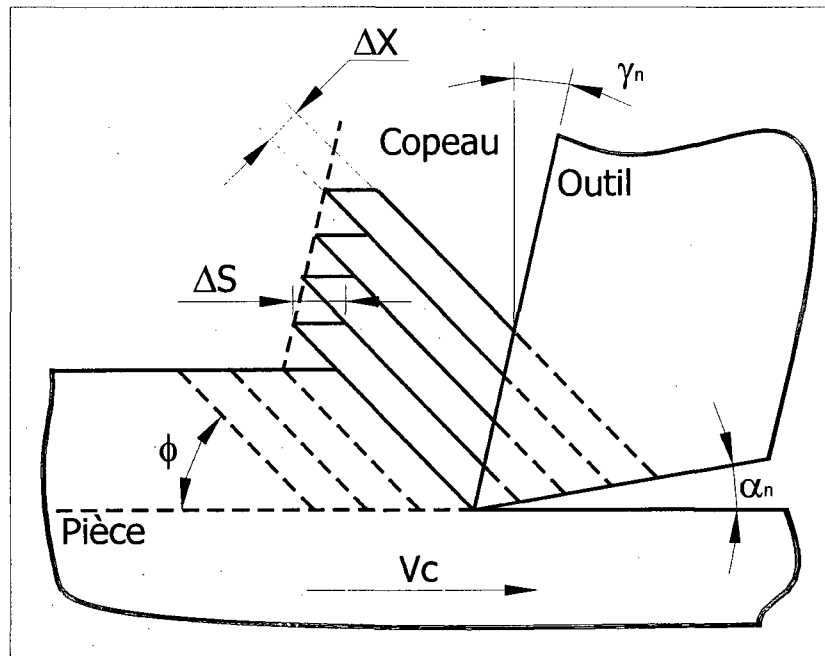
Figure 2.1 Méthode de Merchant pour l'estimation de \bar{\gamma} .
