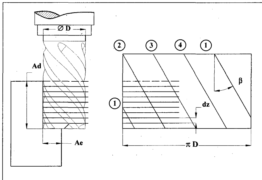
Figure 1.3 Discretisation d'une fraise à quatre flutes 1 .
