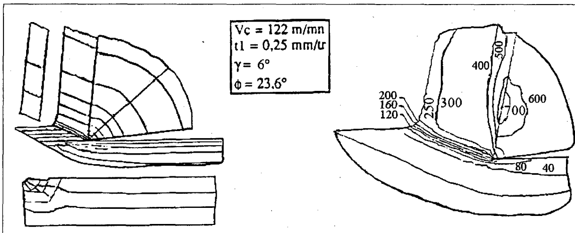
Figure 1.20 Isothermes dans le modèle d'Oxley : Deuxième étude [10].
