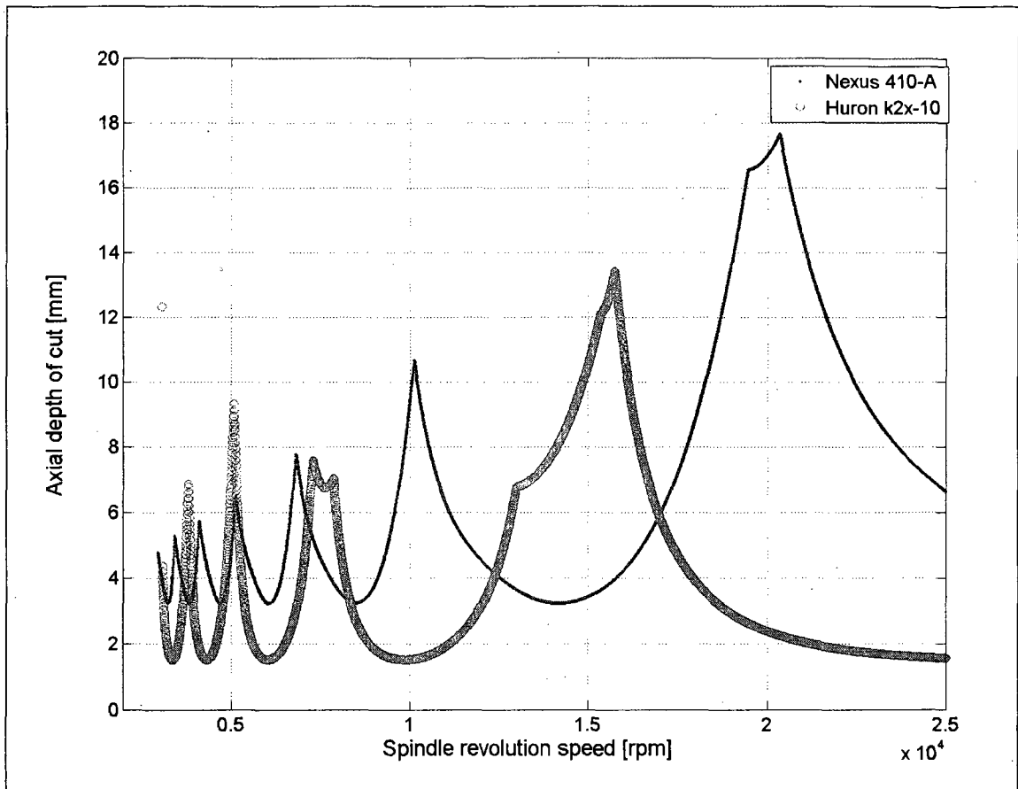
Figure 3.6 Lobes de stabilité pour deux machines outils à commande numérique.
