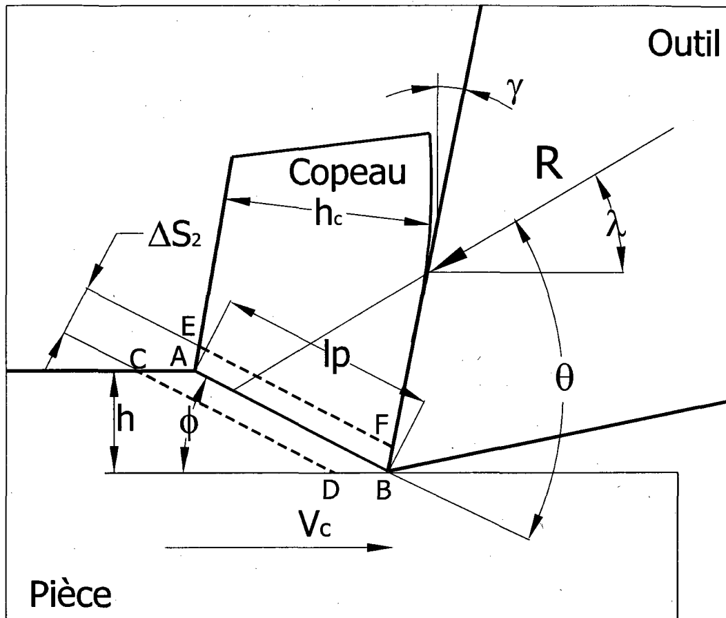
Figure 1.14 Modèle du formation du copeau selon Oxley.
