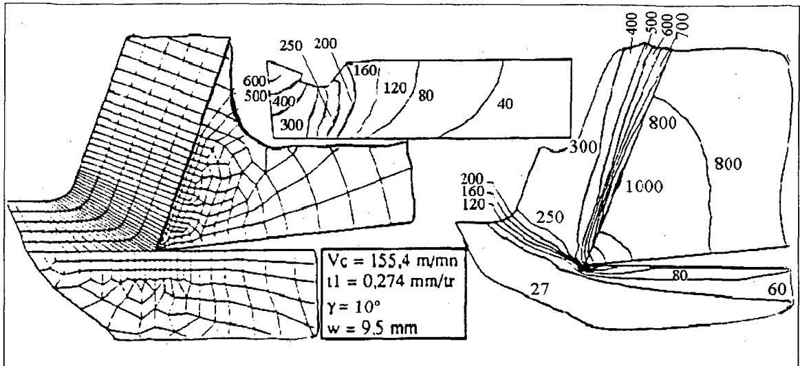
Figure 1.19 Isothermes dans le modèle d'Oxley : Première étude [10].
