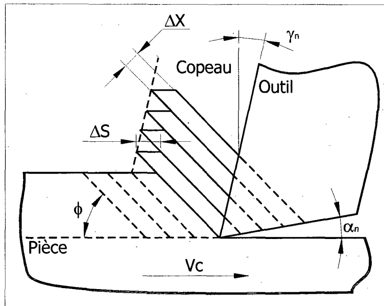
Figure 1.11 Détermination géométrique de \gamma .
