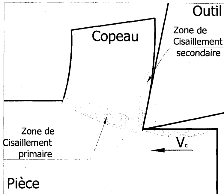
Figure 1.7 Les principales zones de cisaillement.
