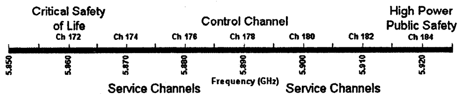
Fig. 1.5. DSRC spectrum band [11].
