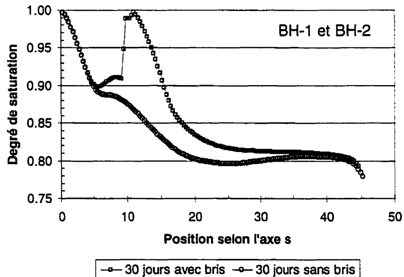
Figure 6.41 : Évolution du S_r calculé au milieu de la couche de rétention d'eau en fonction de la localisation dans la pente ( s=0 correspond au bas de la pente) pour une CEBC avec ou sans bris hydraulique au bas soumise à une période de drainage prolongée de 30 jours
