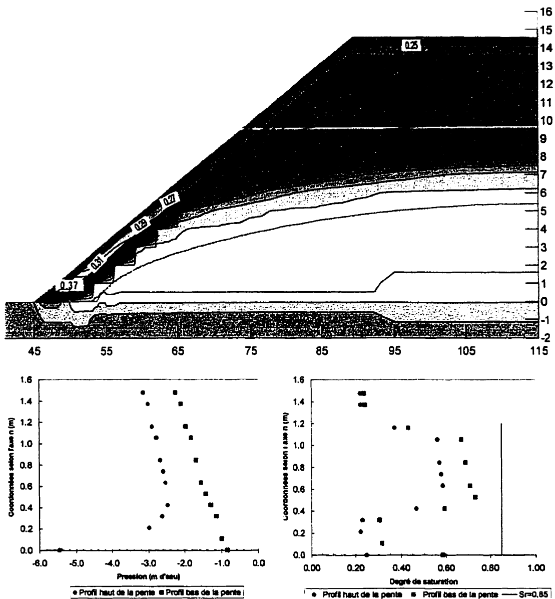
Figure 6.20 : Résultats de la simulation LTA-12 après 60 jours de drainage présentés sous la forme de contours couleurs de la teneur en eau volumique et de profils, pris au haut et au bas de la pente, du degré de saturation et de la succion
