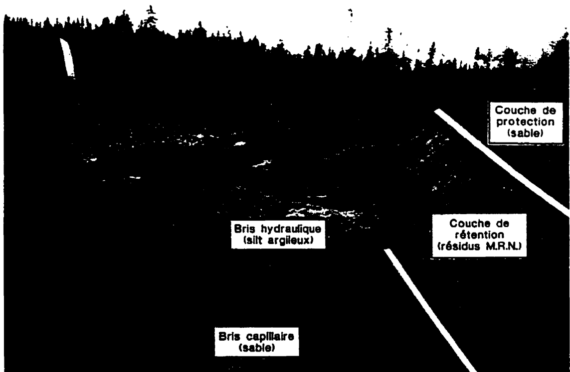
Figure 6.37 : Photographie prise lors de la mise en place du bris hydraulique expérimental placé sur le site LTA (Golder et associés, 1999)
